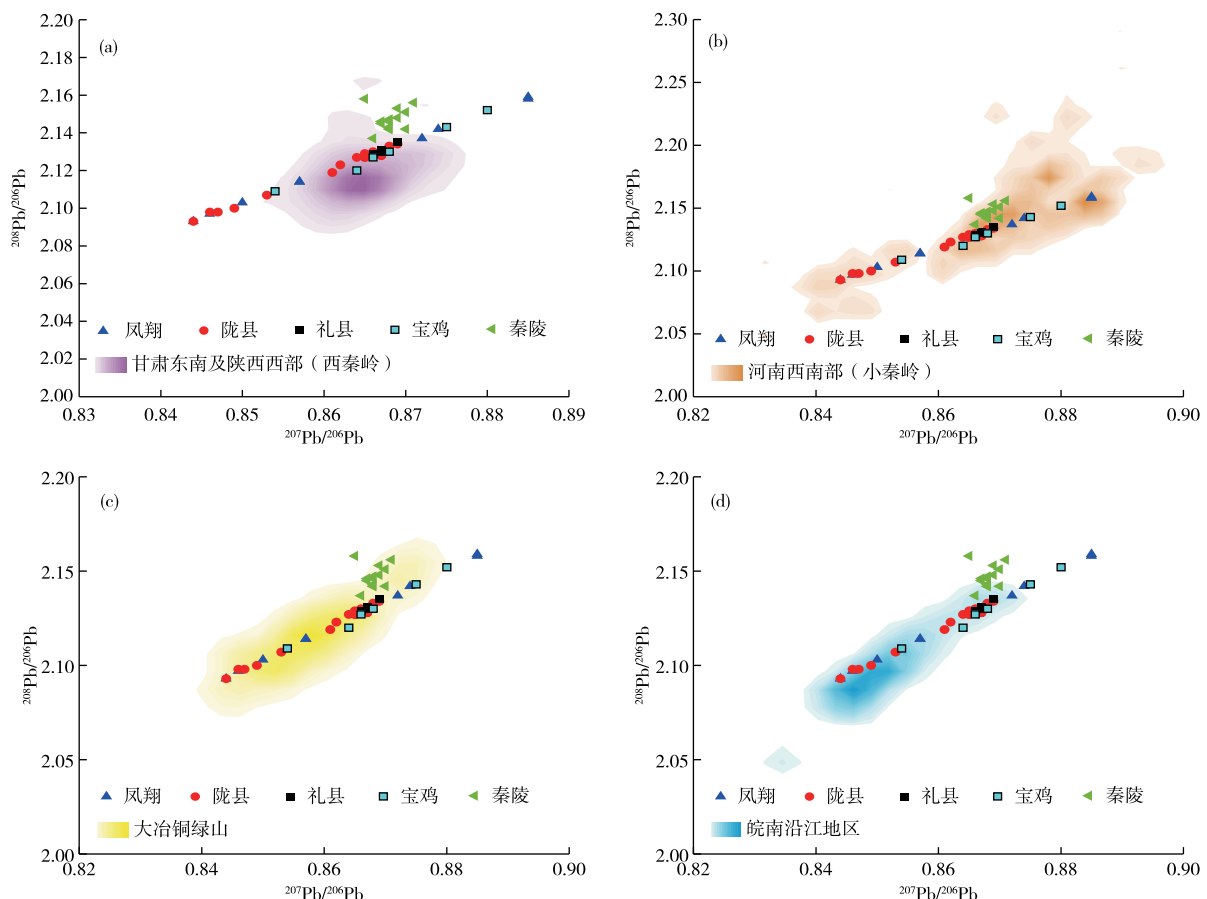
图4 秦国青铜器与各地区矿料铅同位素数据核密度比较图
