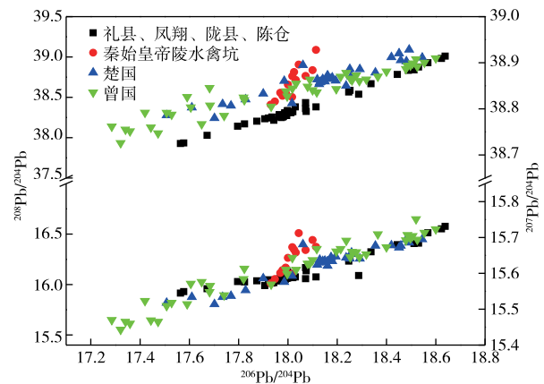
图 3 秦国青铜器铅同位素与楚国、曾国青铜器铅同位素对比
